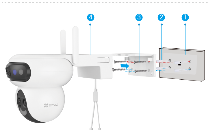
Abb. 2 Wandmontage
