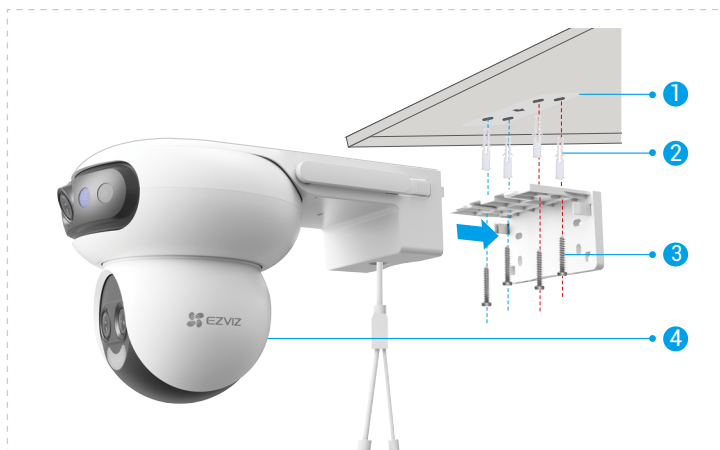
Abb. 1 Deckenmontage
